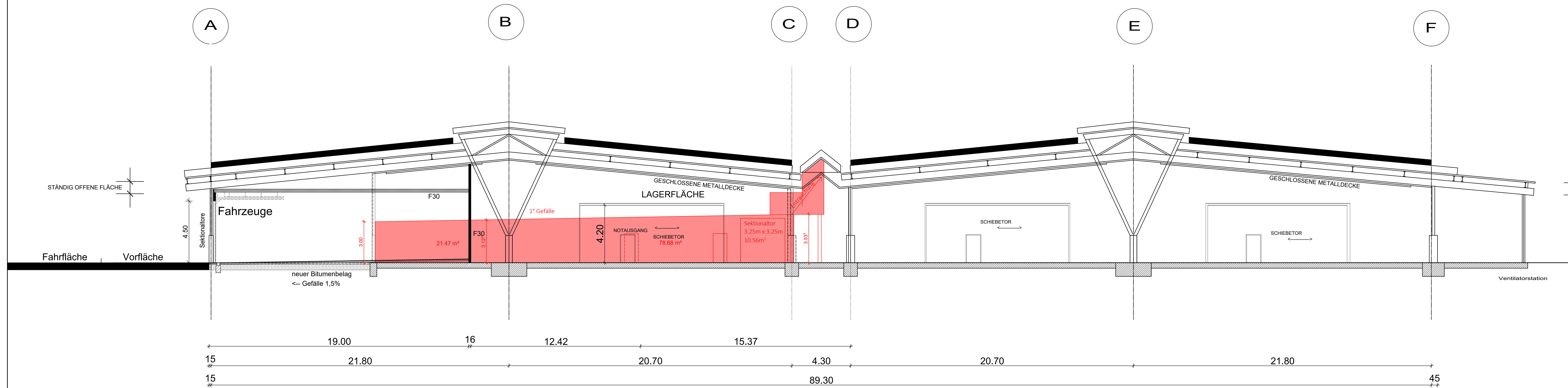
SCHNITT 1-1
